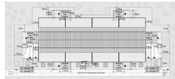
Рис. «Основные параметры места размещения нестационарного торгового объекта для торговой галереи»
