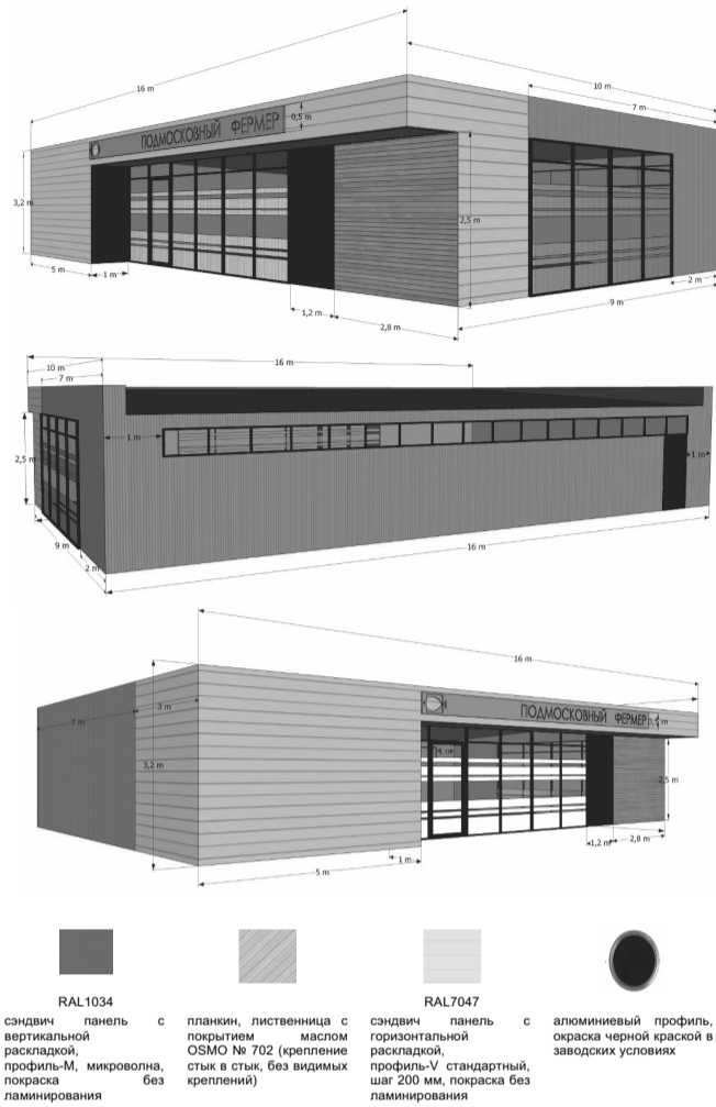
Рис. «Допустимые варианты габаритов элементов специализированного павильона при планировании установки»
